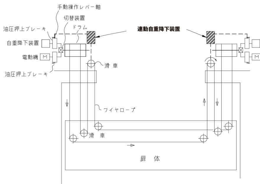
【 連動自重降下機構 概略図 】
